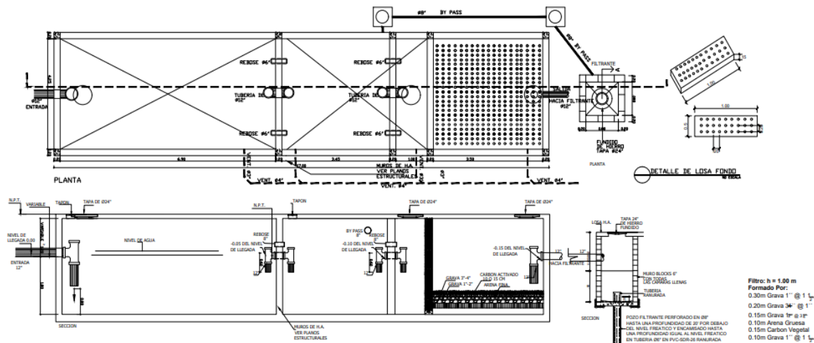
Detalle Cámara Séptica con filtro Matadero Municipal
