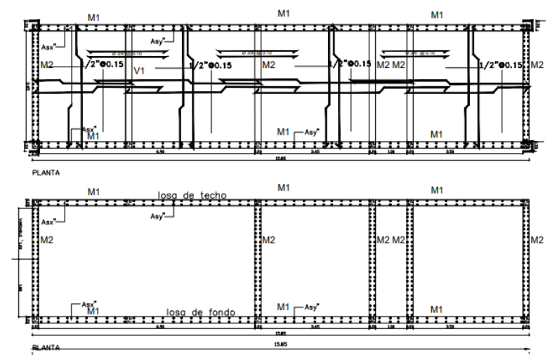
Detalle UND Tratamiento de aguas residuales Matadero Municipal
